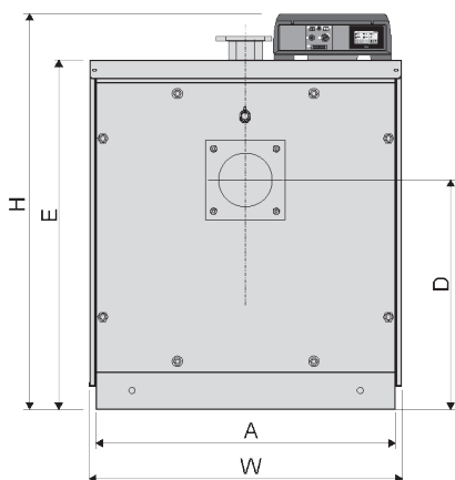
VISTA POSTERIORE
