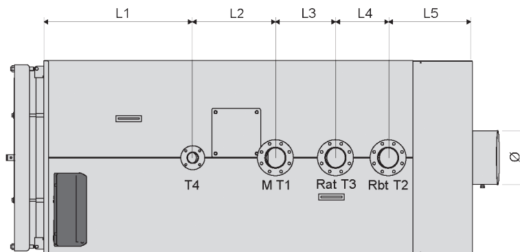
VISTA SUPERIORE
