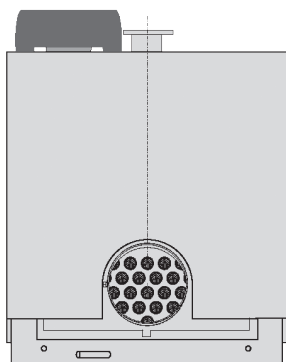
VISTA POSTERIORE
